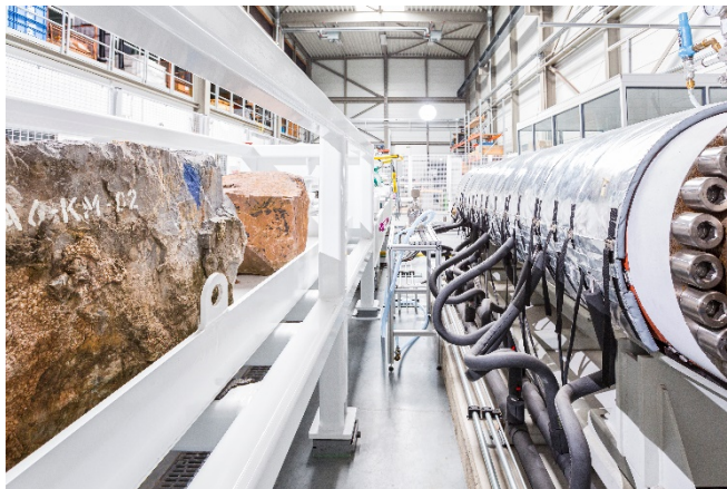
Abb. 3 Wie verhält sich ein Gestein bei extremem Druck? Mit dem Fraunhofer-IEG-Teststand kann diese Frage nun deutlich schneller und ökonomischer beantwortet werden.
