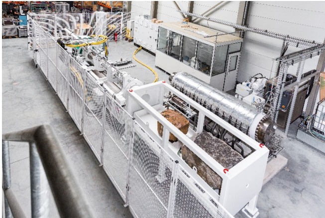
Abb. 2 Testen für den Ernstfall: Die match.BOGS simuliert Bedingungen, die in mehreren Tausend Metern vorherrschen.
